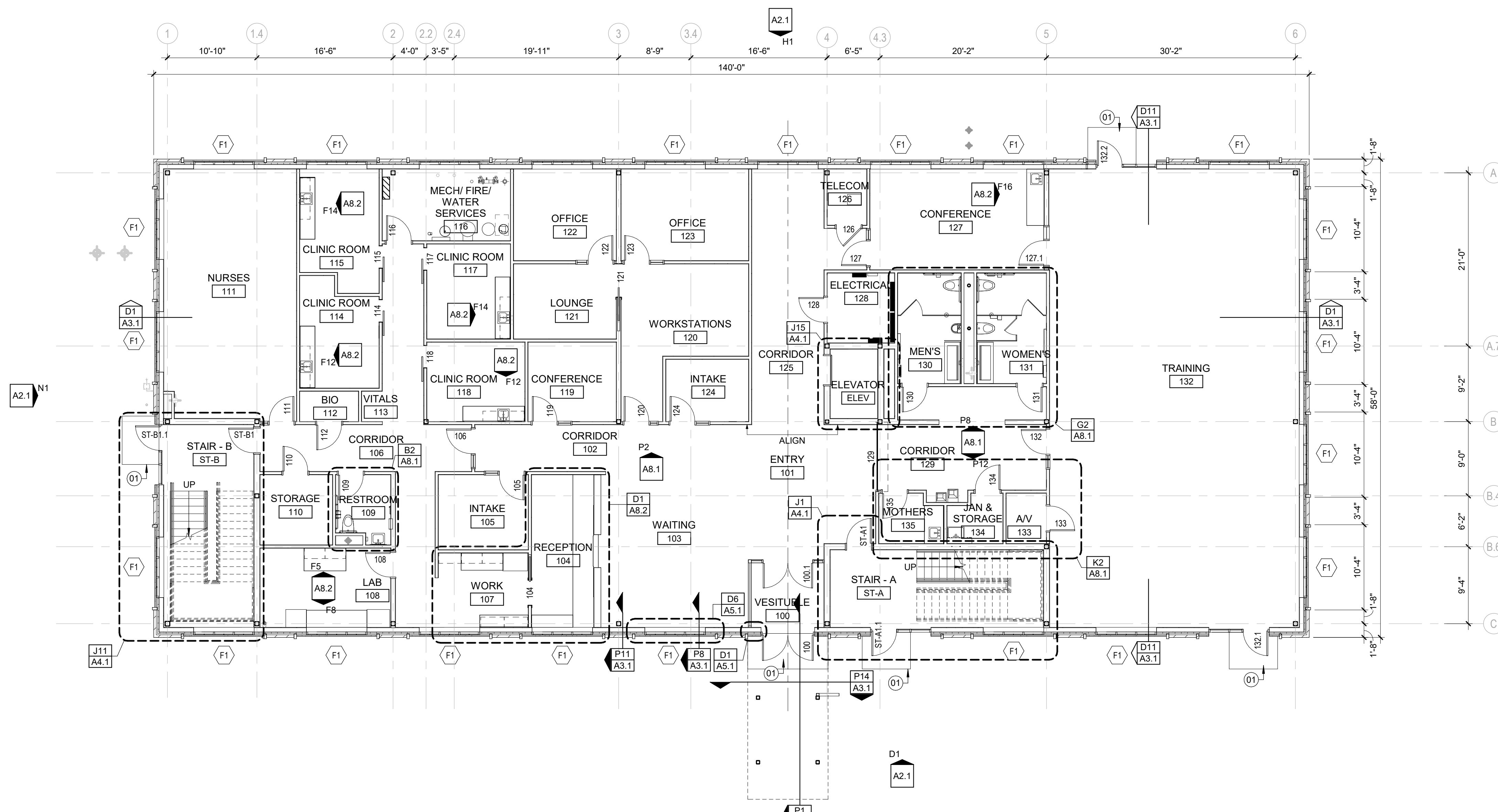
G2 FLOOR PLAN - LEVEL 02 A1.1 SCALE: 1/8" = 1'-0"
