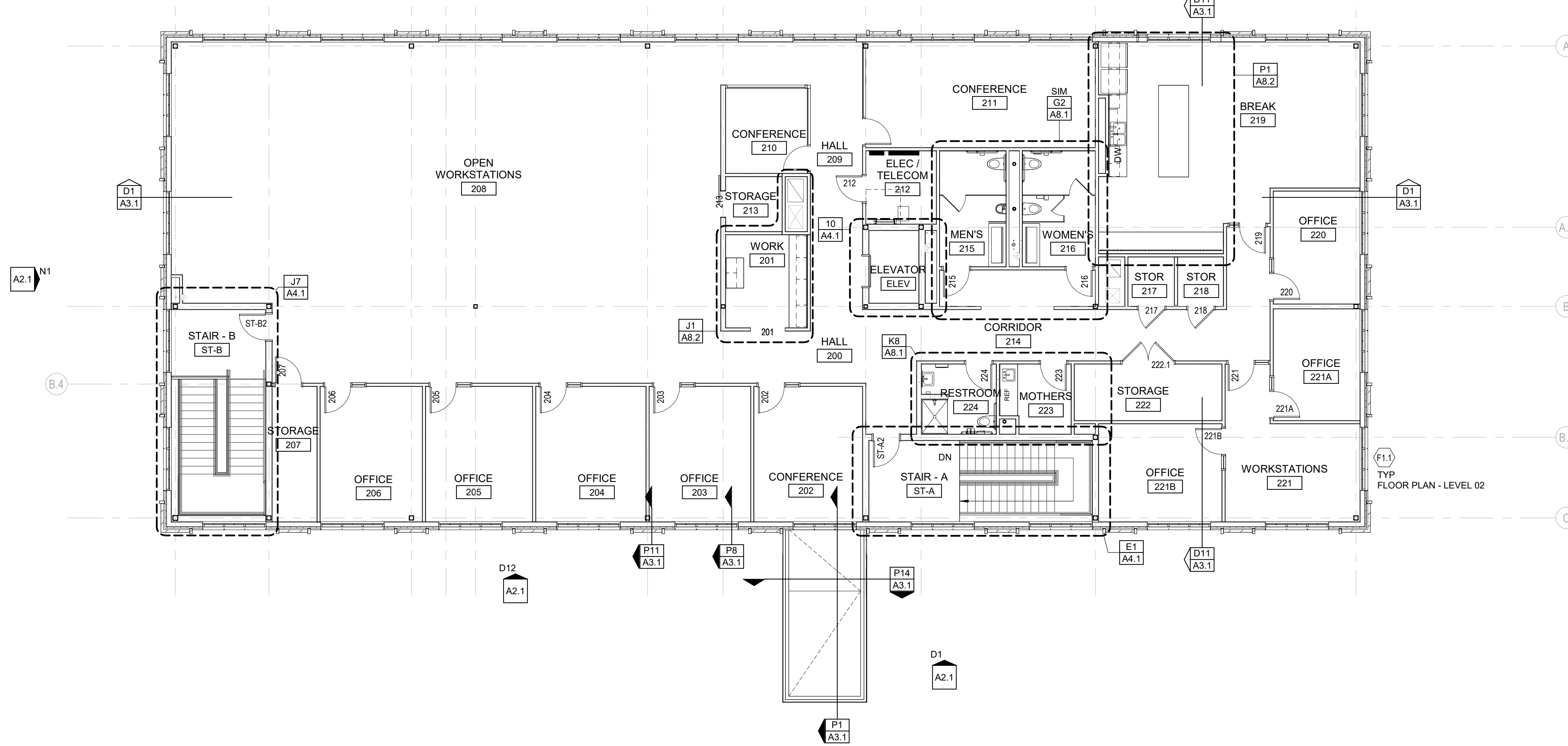
G2 FLOOR PLAN - LEVEL 02 A1.1 SCALE: 1/8" = 1'-0"
